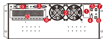
10 kVA (S) (3:1)
